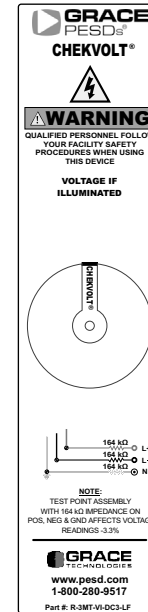
Flange Label* (R-3MT-VI-DC3-LF)
