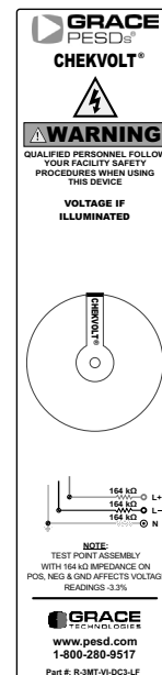
Étiquette de la bride* (R-3MT-VI-DC3-LF)
